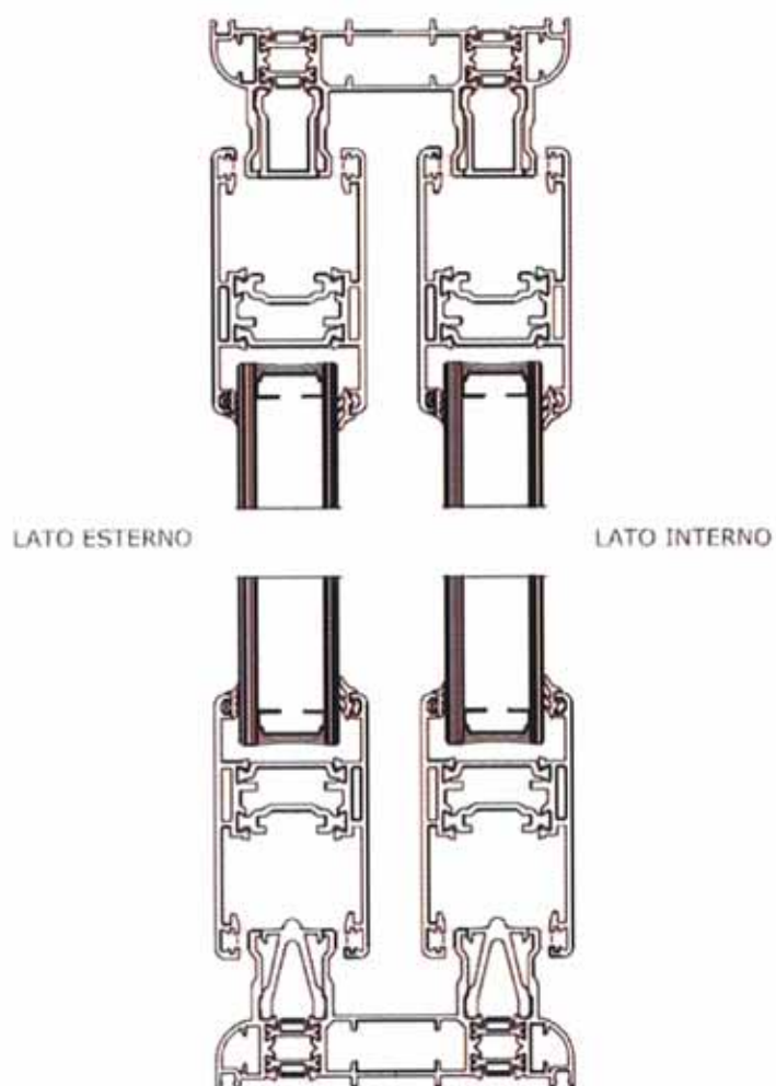
Fig.3 - Sezione orizzontale.
