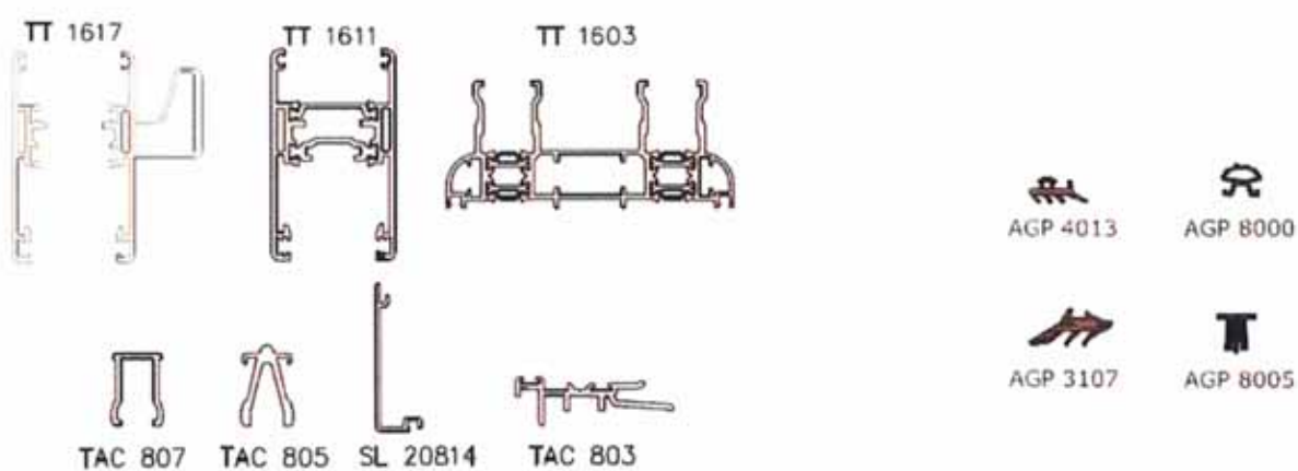
Fig.4 - Particolari.
