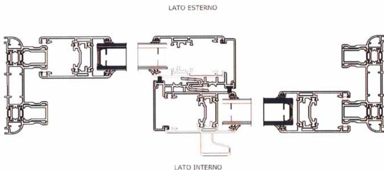
Fig.2 - Sezione verticale.
