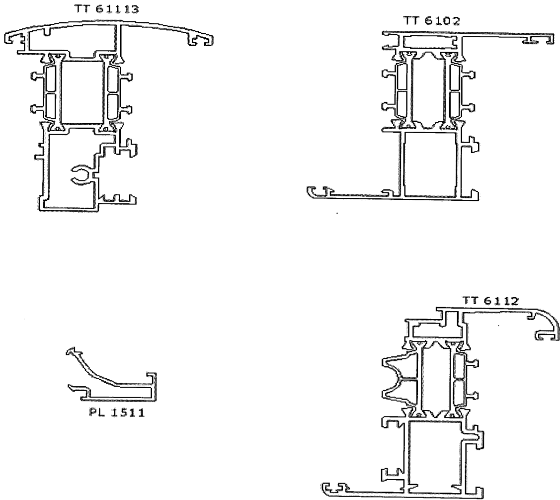
Fig.4 – Sezioni profilati.
