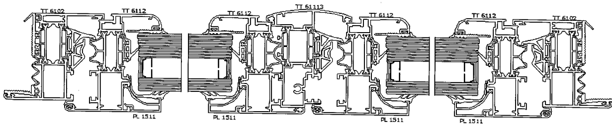
Fig.2 – Sezione orizzontale.
