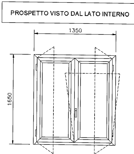
Fig.1 – Prospetto del campione sottoposto a prova.
