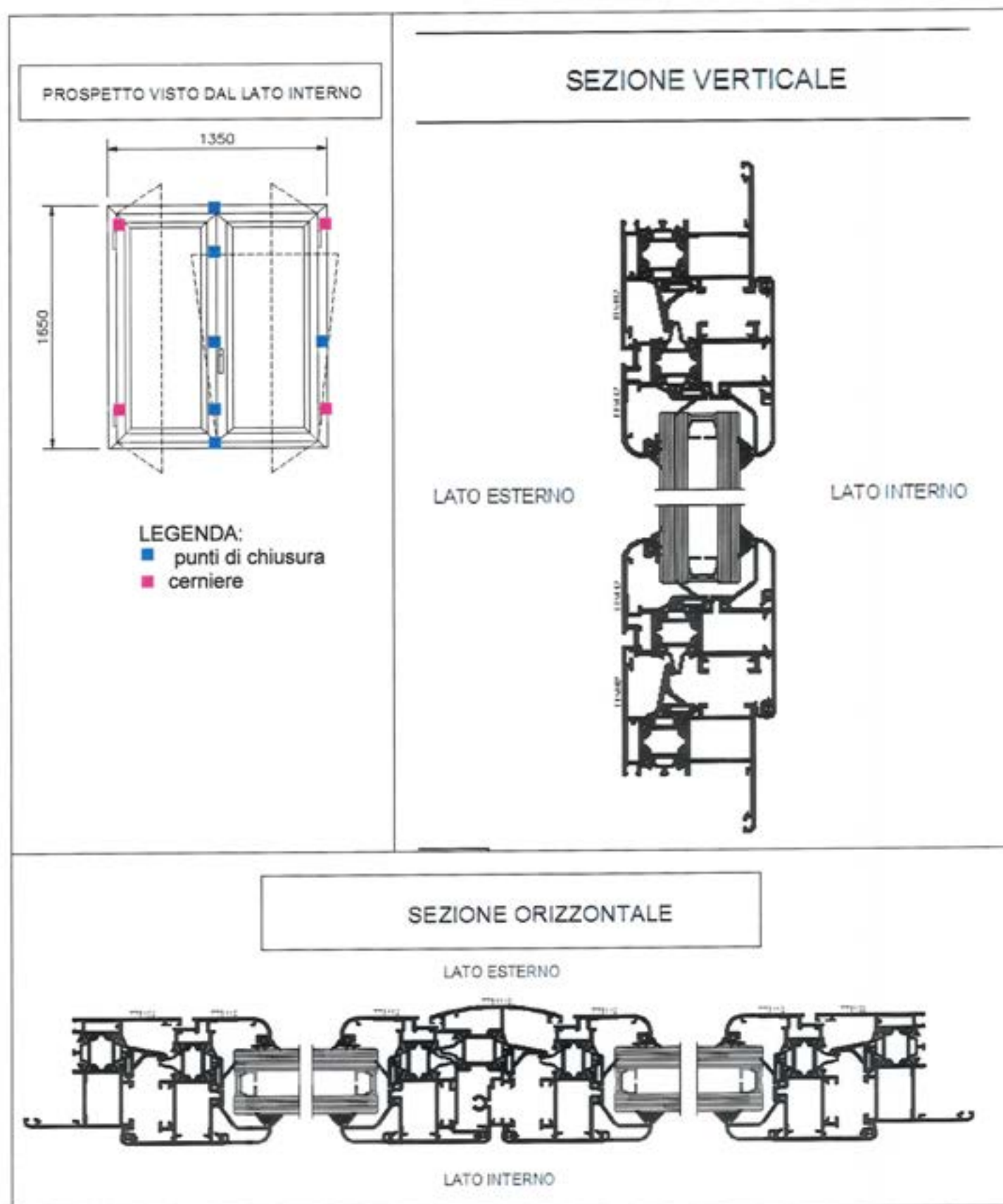
Fig. 1: Prospetto vista interna con indicazione dei punti di chiusura e sezioni orizzontale e verticale del campione pervenuto e sottoposto a prova (dimensioni nominali dichiarate, espresse in mm)
