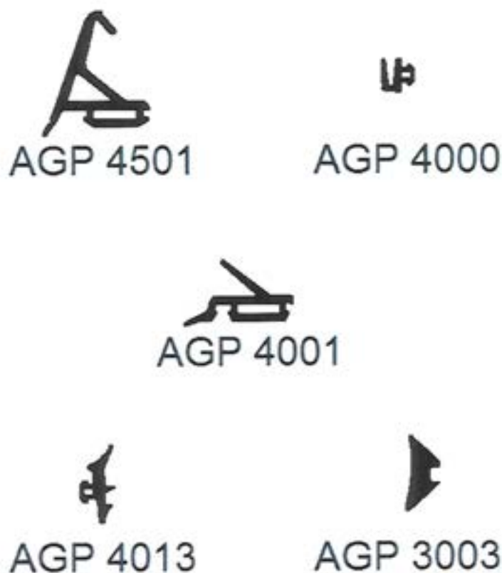
Fig. 3: Sezioni delle guarnizioni del campione pervenuto e sottoposto a prova
