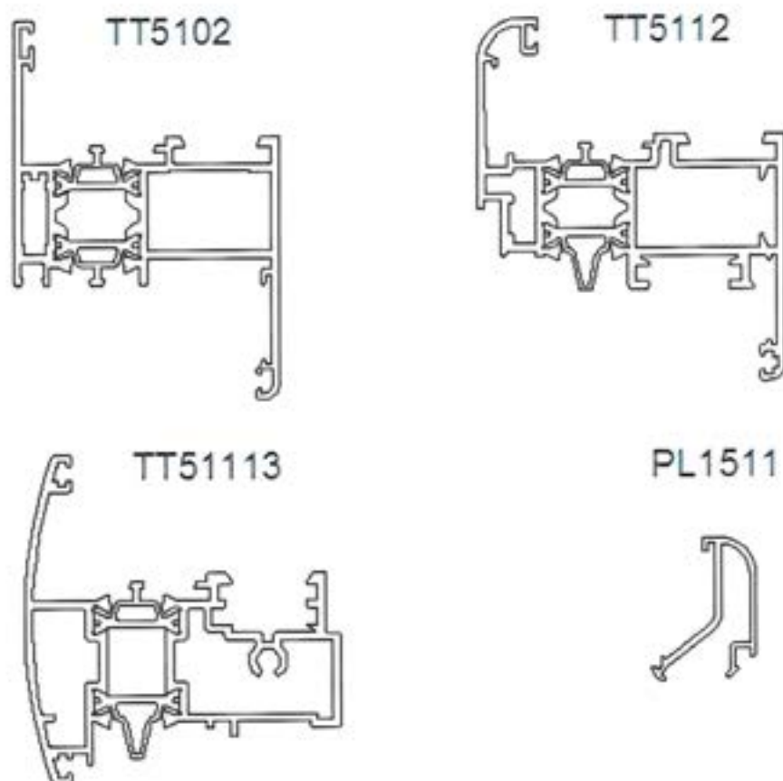
Fig. 2: Sezioni dei profilati e del taglio termico del campione pervenuto e sottoposto a prova
