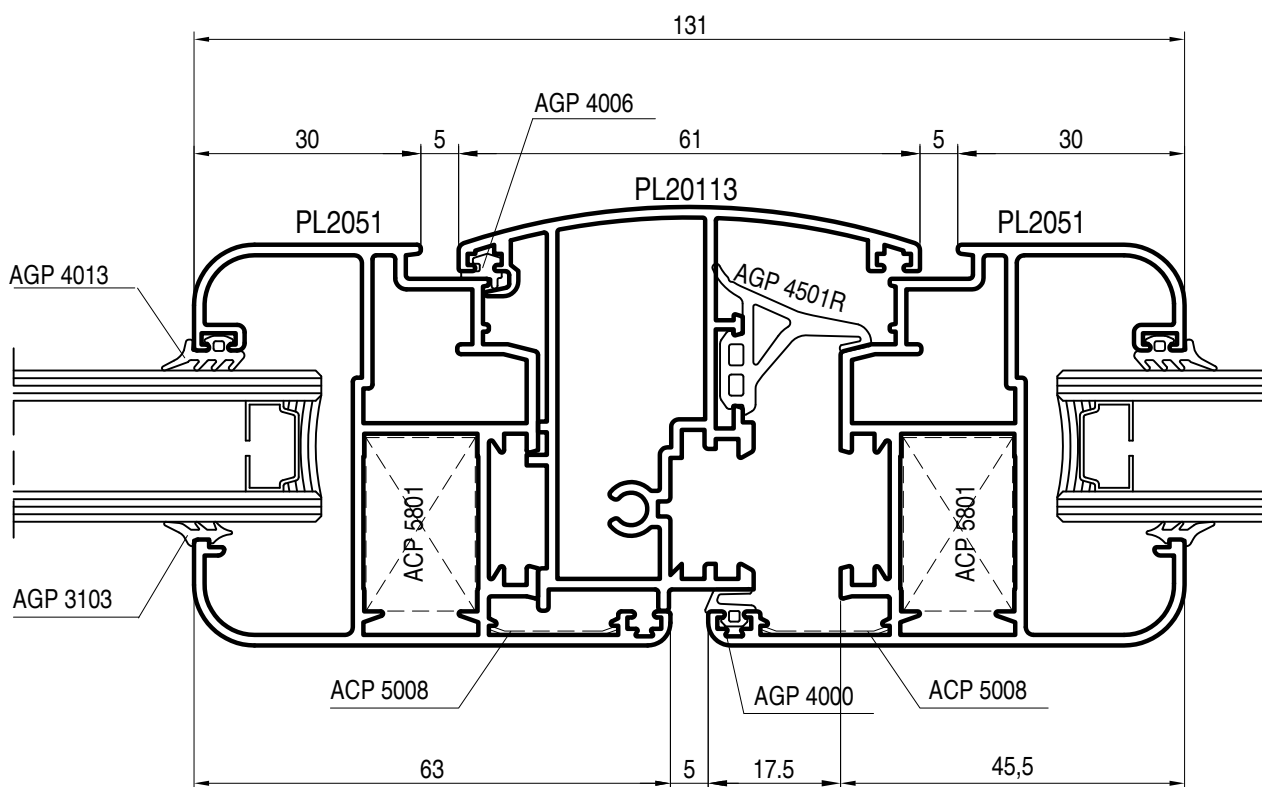
apertura interna - battente - nodo centrale
