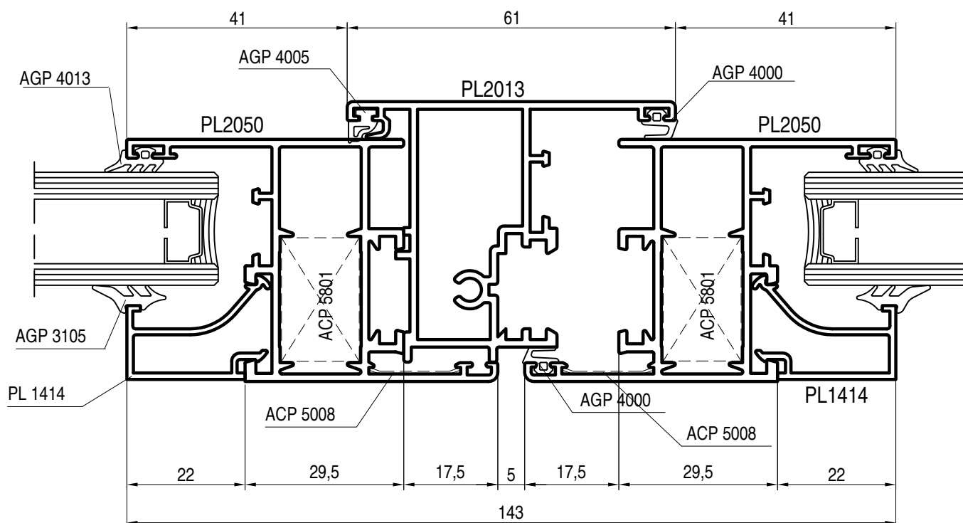
apertura interna - battente - nodo centrale
